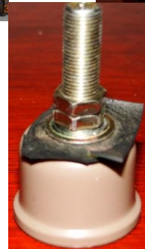
Fig. 9. Detalhes da válvula de pneu de bicicleta preso no “cap”.
