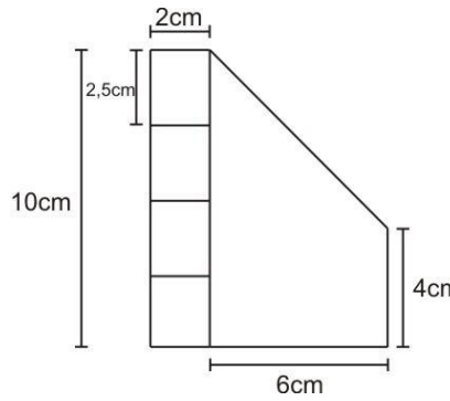
Fig. 2. Dimensões e formato da aleta
